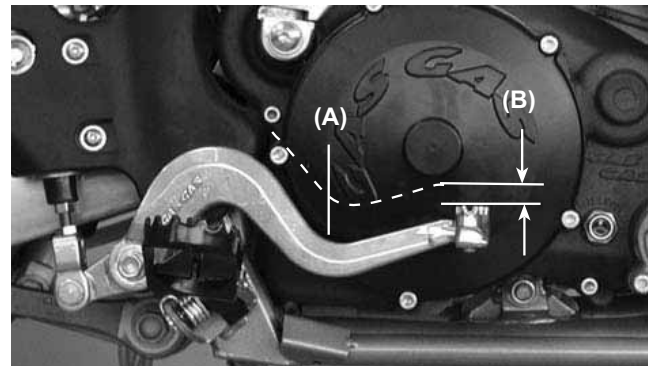
(A). Levier du frein. (B). 10 mm de jeu.
