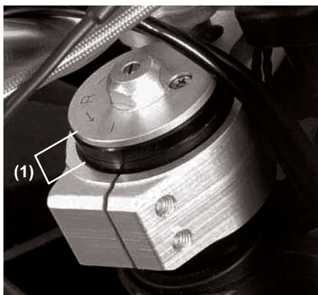
(1). Position der Federungsplatte.
