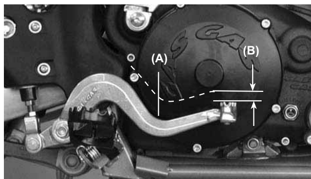
(A). Pedale freno. (B). 10 mm di gioco.
