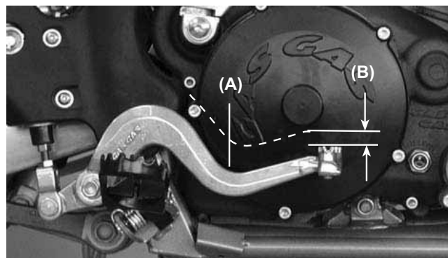
(A). Pedal freno. (B). 10 mm de juego.
